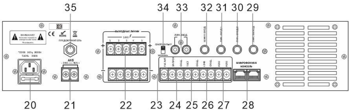
Рис. 1.3. Задняя панель
