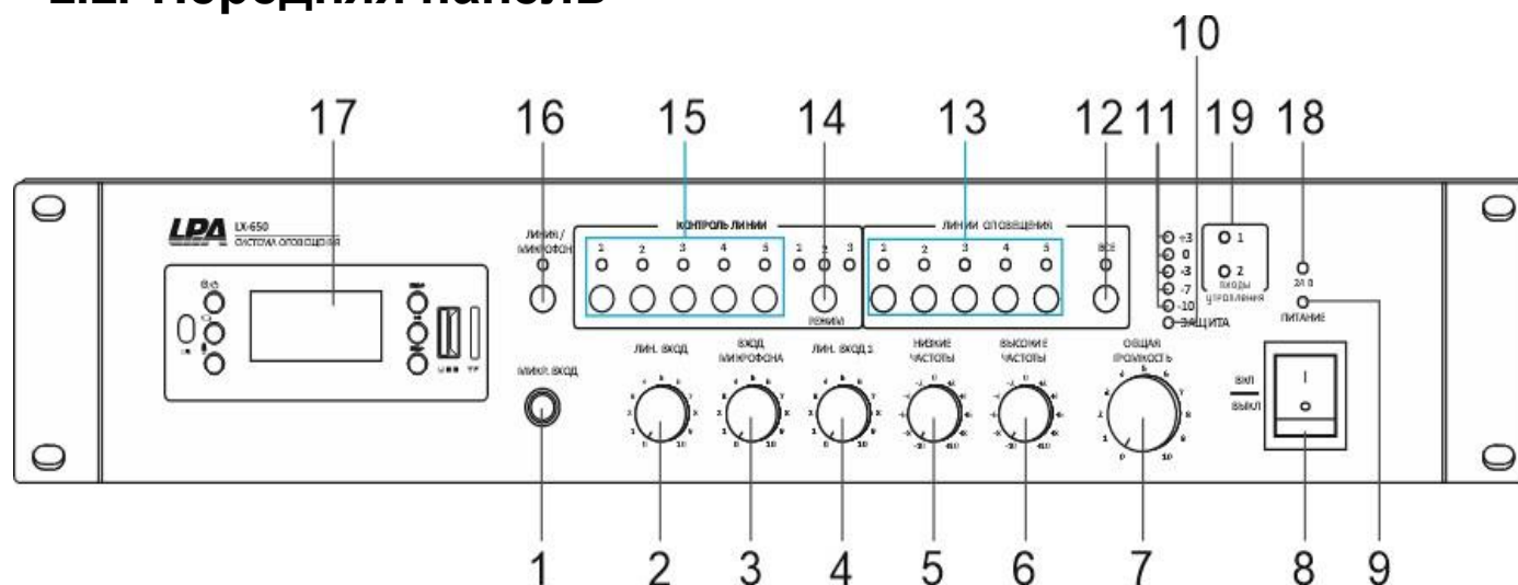
Передняя панель
